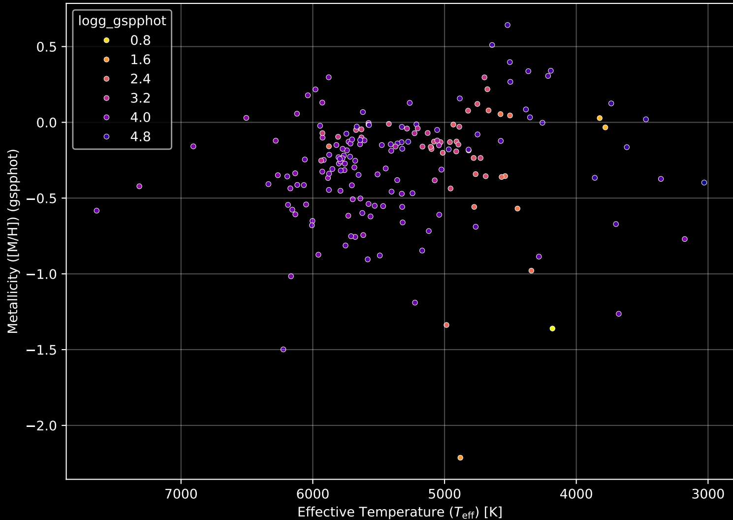
APOGEE DR17 Field: [286-36-O_TESS] Stellar Population Parameters (n= 182)
